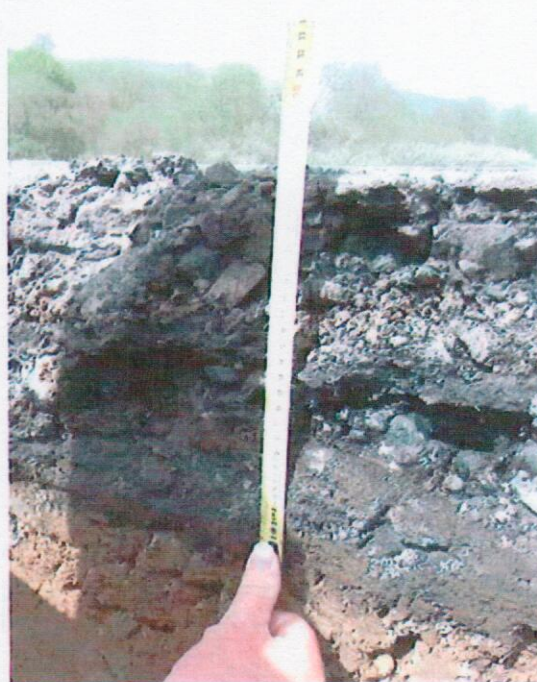
Obr. 6 Konštrukcia pôvodnej vozovky
